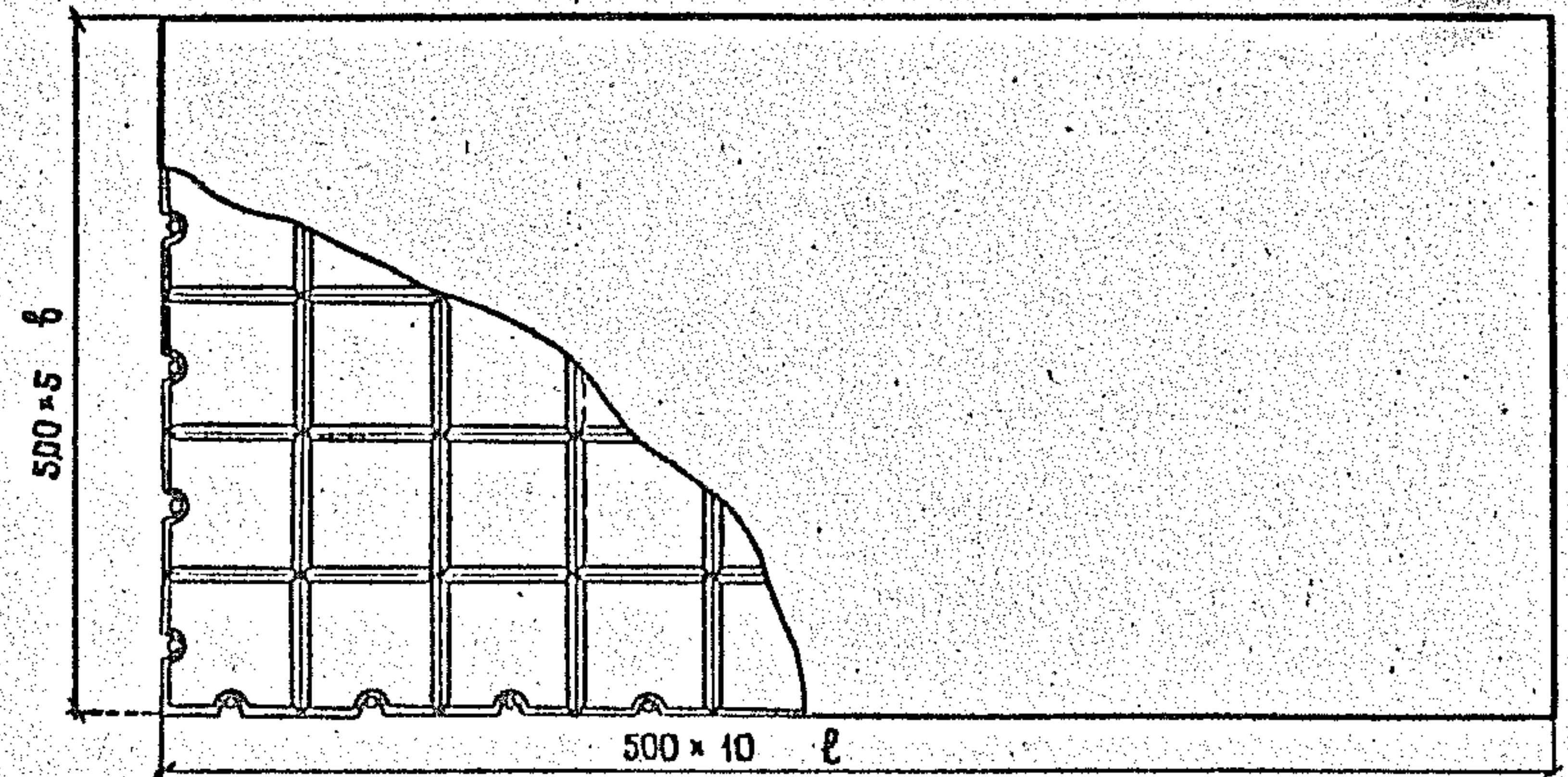
ГИБКАЯ ЖЕЛЕЗОБЕТОННАЯ ПЛИТА ПГ-10; ПГ-12; ПГ-15
