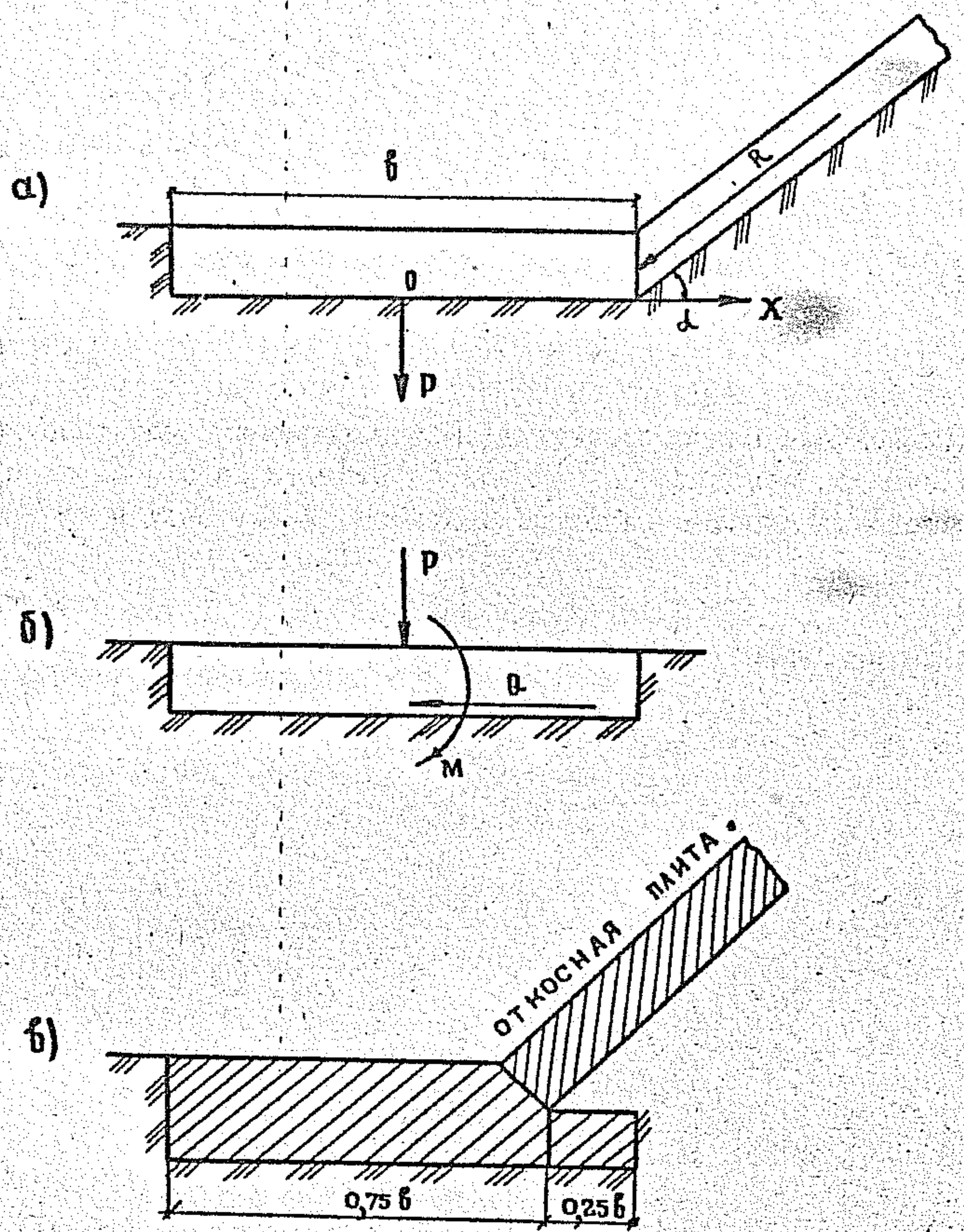
а) СХЕМА ДЕЙСТВУЮЩИХ СИЛ б) РАСЧЕТНАЯ СХЕМА ПЛИТЫ в) СХЕМА РАЦИОНАЛЬНОГО ПРИМЫКАНИЯ ОТКОСНОЙ ПЛИТЫ К УПОРНОЙ ПРИЗМЕ
