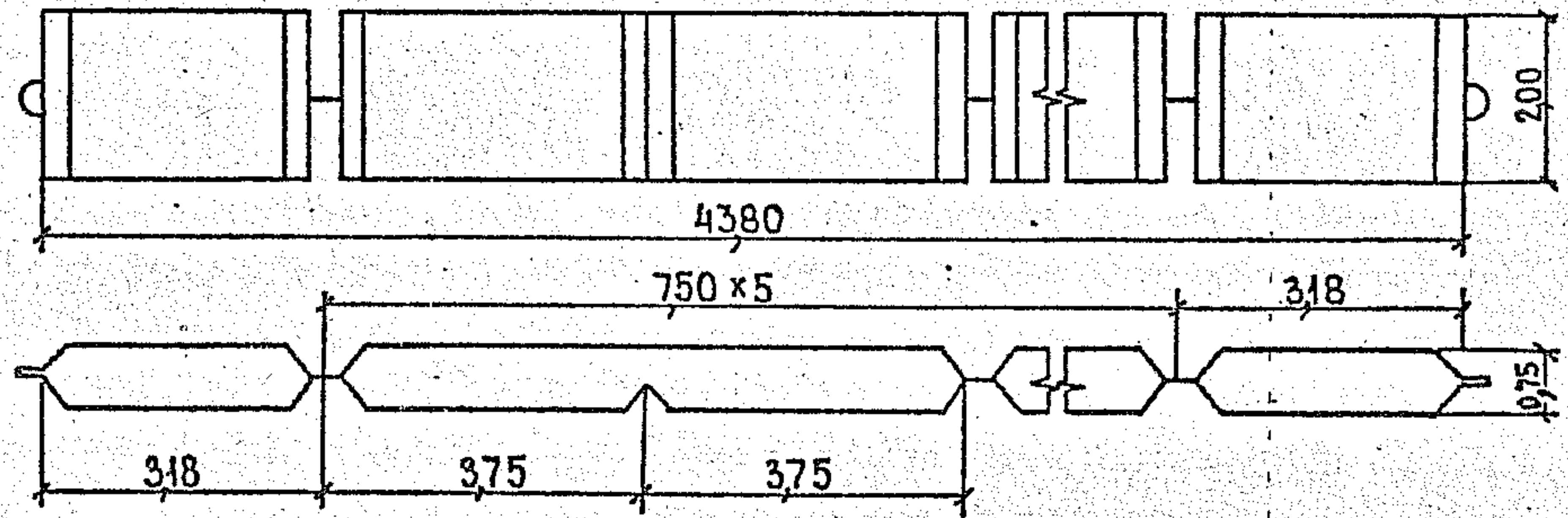
ГИБКАЯ ГИРЛЯНДА
