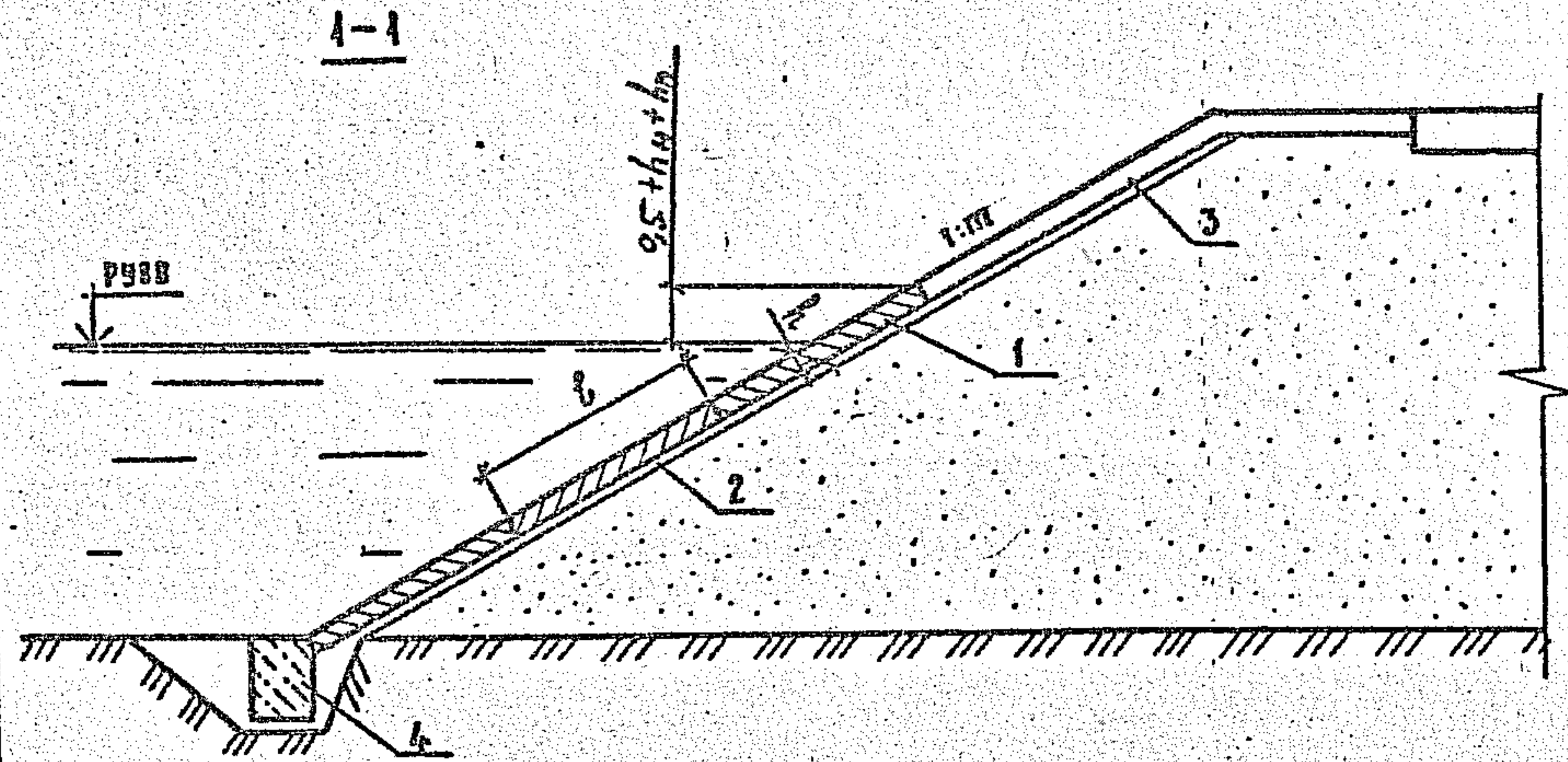
h_n - высота наката ветровых волн, h_p - высота подпора воды.
