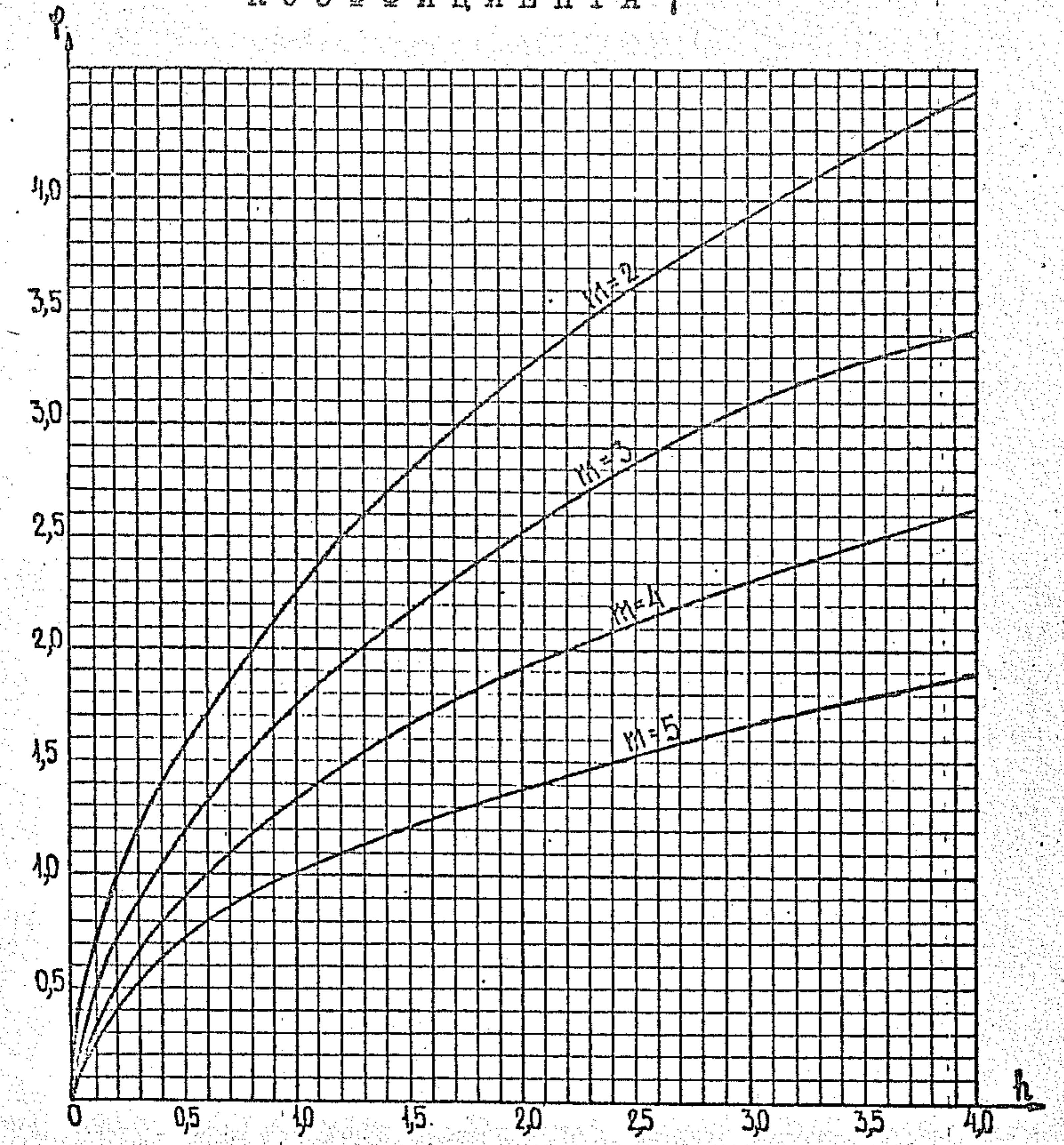
ГРАФИК ДЛЯ ОПРЕДЕЛЕНИЯ КОЭФФИЦИЕНТА \psi
