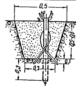
Поперечный разрез
