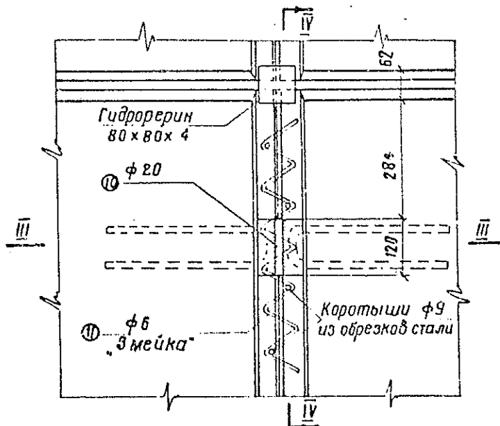
План стыка „Б“
