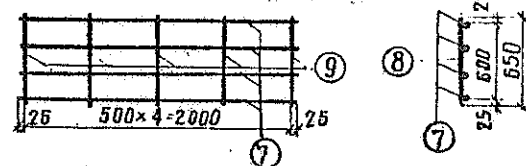
Спецификация арматуры
