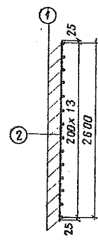
Каркас для омоноличивания К-2
