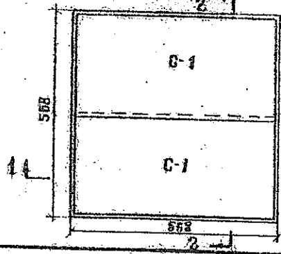
План расположения арматурных сеток
