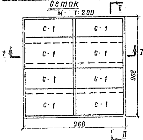
План расположения арматурной
