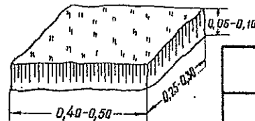
Штычный дёрн
