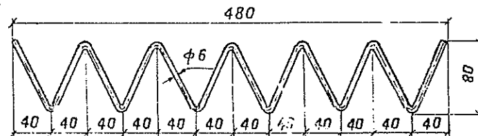
Спецификация арматуры на стык „Б“
