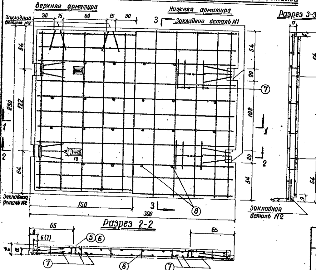
План расположения арматурных сеток и закладных деталей
