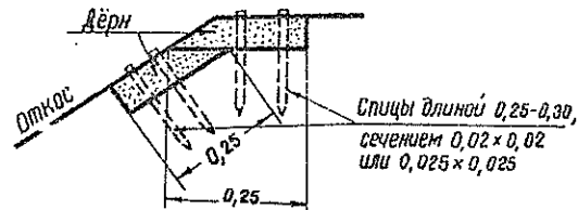
Штычный дёрн
