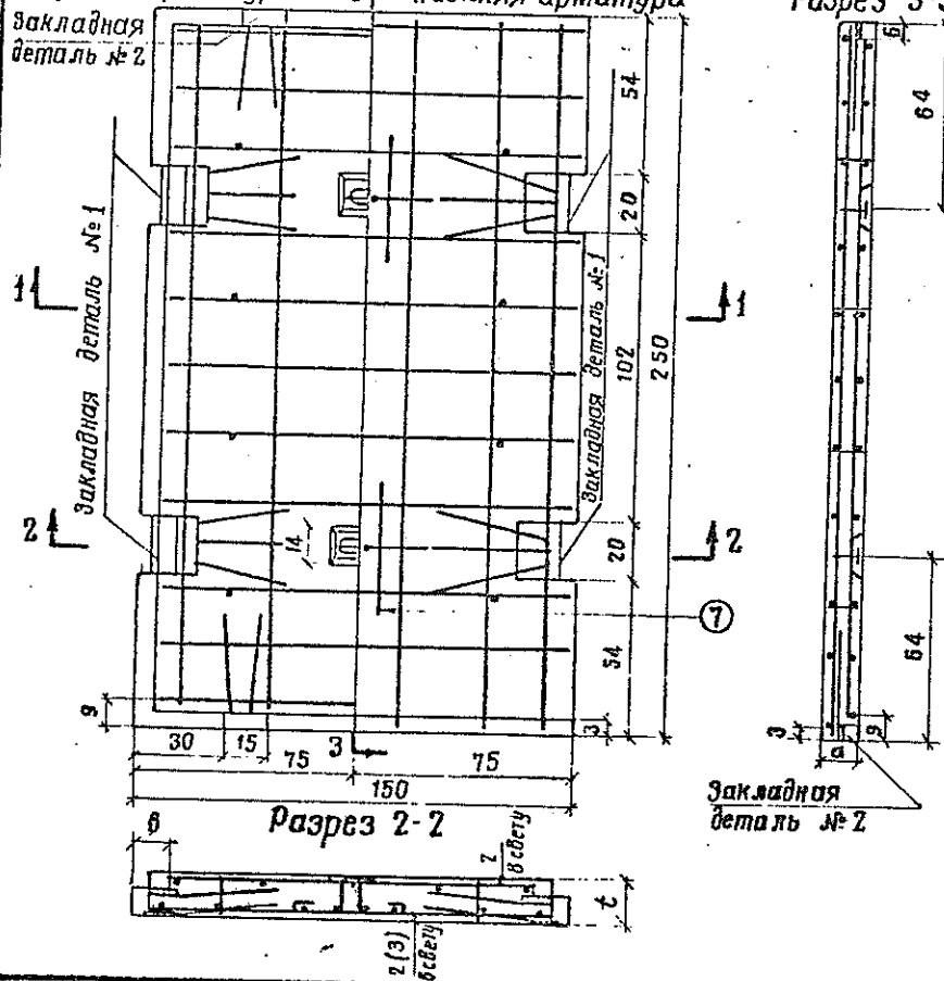
План расположения арматурных сеток и закладных деталей Верхняя арматура 3 — Нижняя арматура
