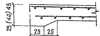
Конструкции креплений откосов земляного полотна
