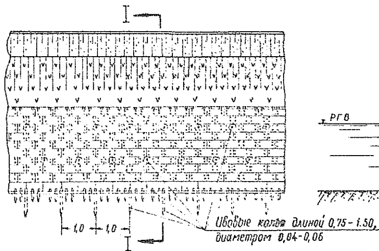
Вид откоса
