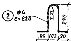
Монтажная петля
