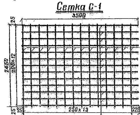
План расположения арматуры
