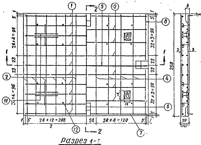
Нижняя сетка
