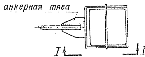
План
