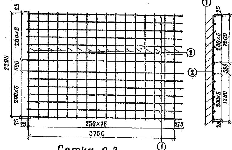
Сетка С-2
