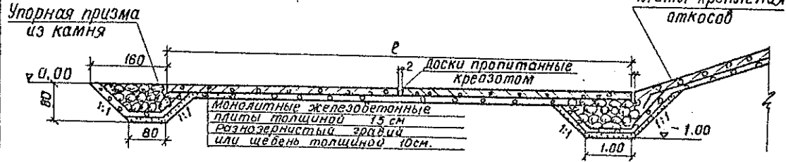
Разрез 1-1
