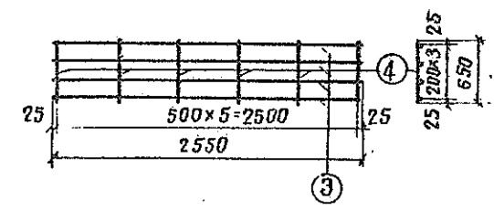
Каркас для омоноличивания К-2
