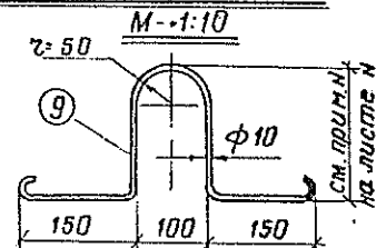
Монтажная петля
