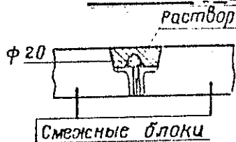
Сечение I-I
