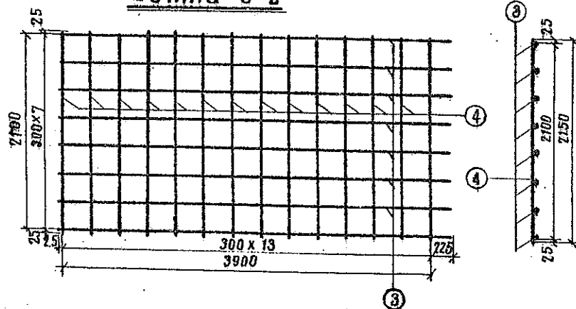
Сетка С-2
