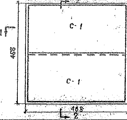
План расположения арматурных сеток
