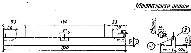
Армирующие плиты
