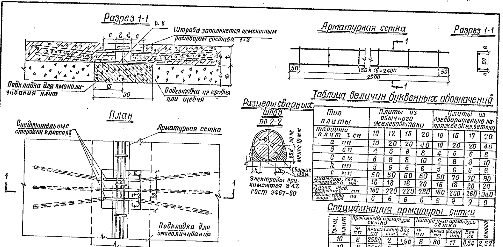
Расход материалов для омоноличивания плит (на 1 п.м.ш.б.а)
