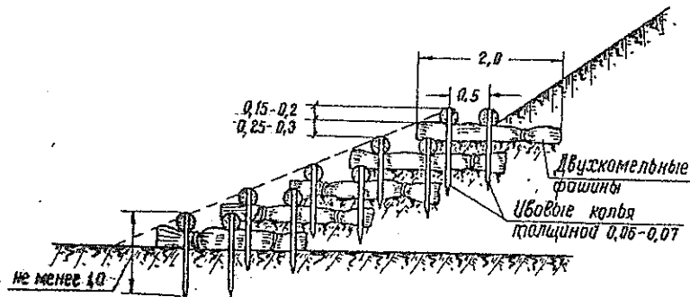
Поперечный разрез
