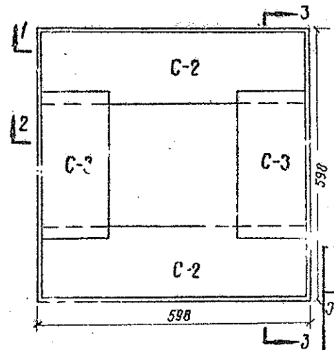
План расположения арматурных сеток
