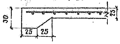
Зуб для нижней плиты М 1:25
