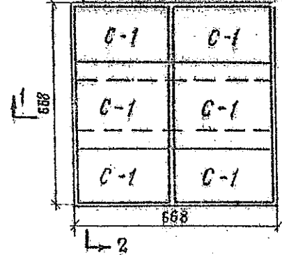
План расположения арматуры
