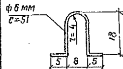
Монтажная петля
