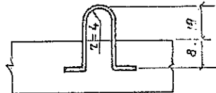
Крепление монтажной петли
